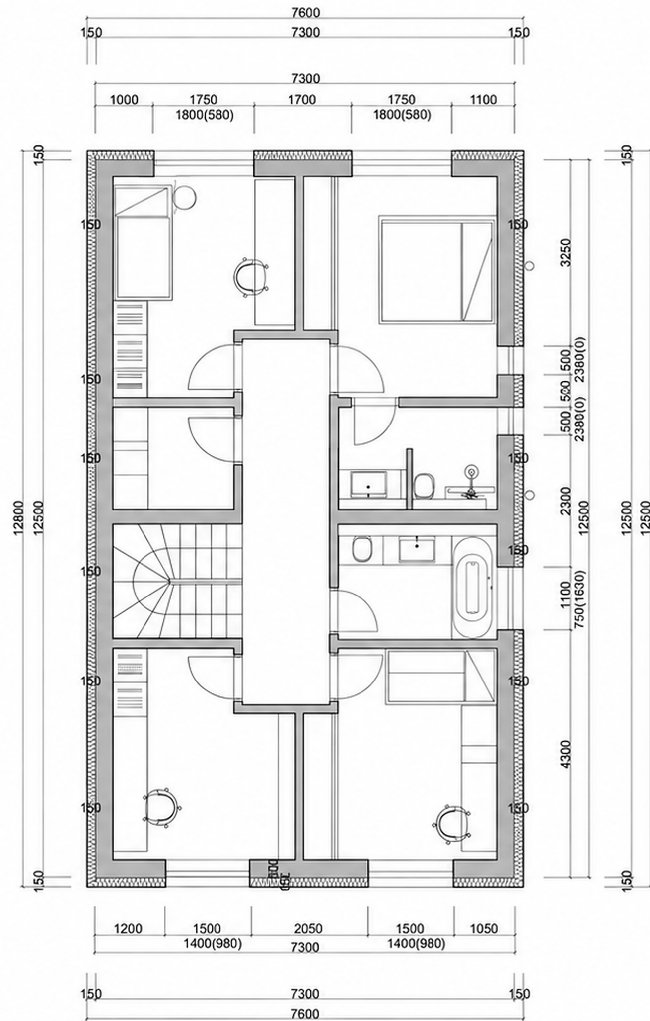
PÔDORYS 2. NP
